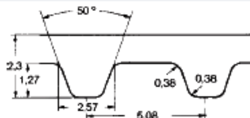
CENTRO DOS DENTES DENTES TRAPEZOIDAIS
